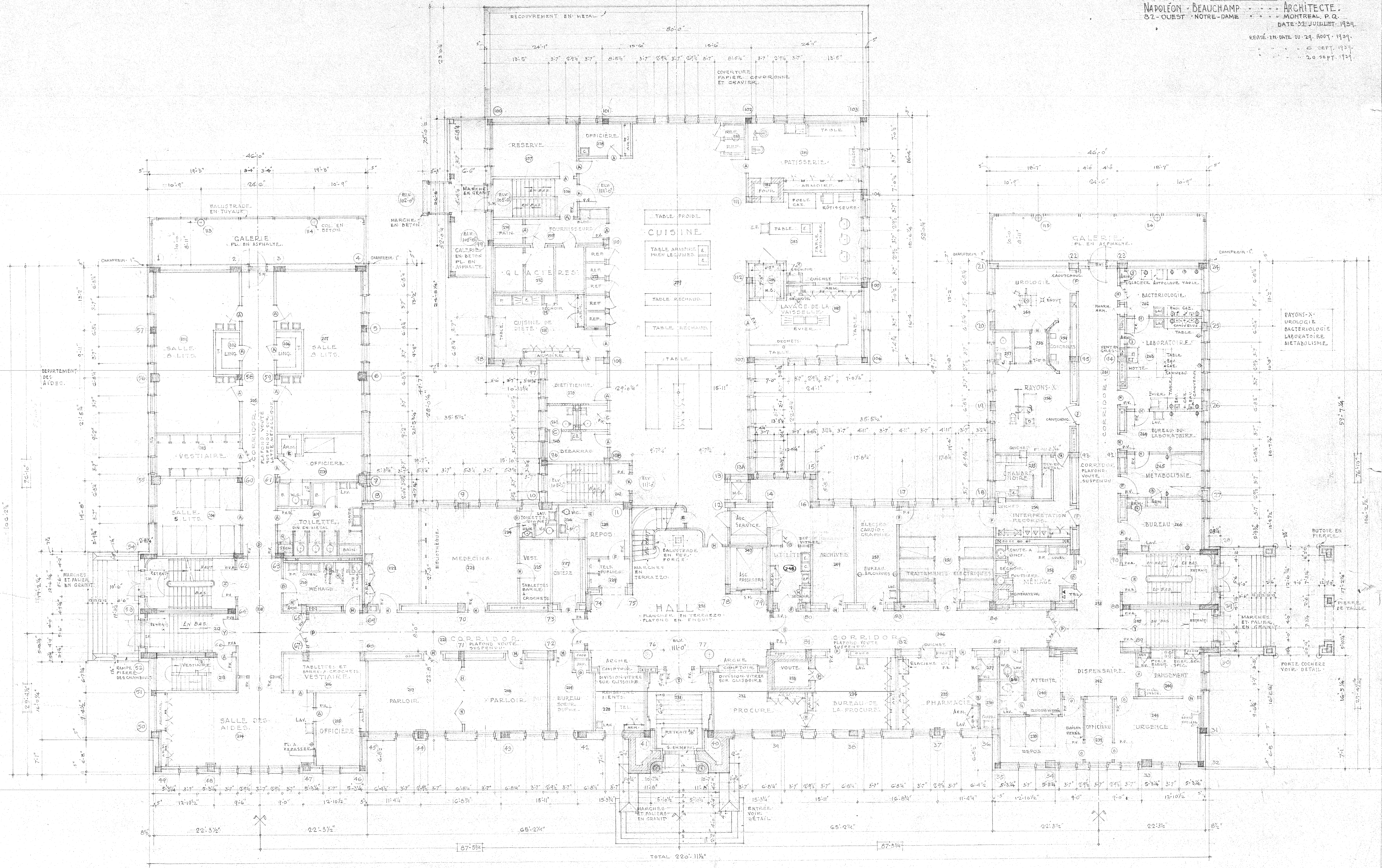
PLAN DU DEUXIEME ETAGE - ELEVATION - IIII - 0
